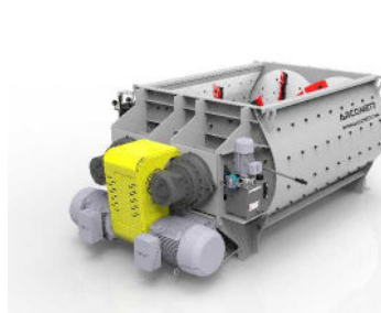
Mezcladora doble eje - MDE
