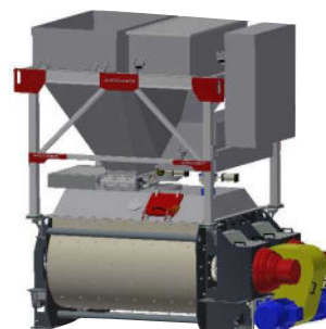
Conjunto dosificación y mezcla
