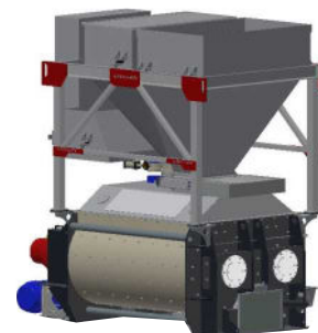
Conjunto dosificación y mezcla
