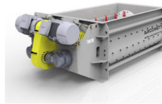
Mezcladora continua - MDC
