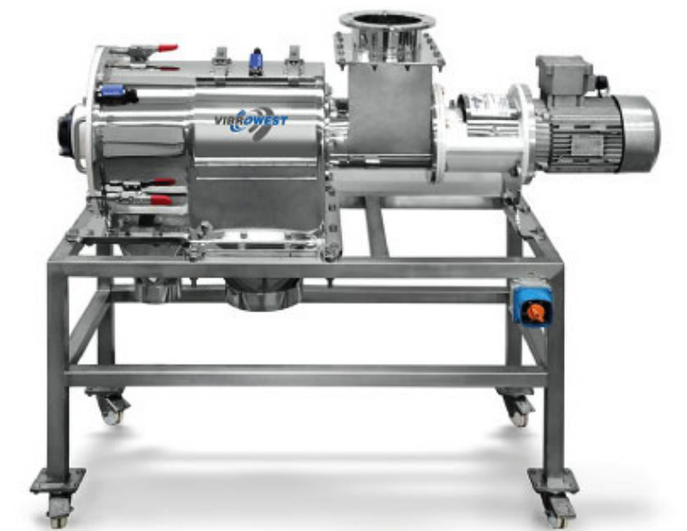
Criba centrífuga Turbowest
